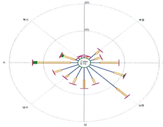
그림 2. 서구지역 바람장미 (주풍향 : 남동풍 계열, 일 평균풍속 : 3.3m/s)
