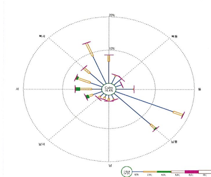
그림 2. 서구지역 바람장미 (주풍향 : 남동풍 계열, 일 평균풍속 : 1.9m/s)
