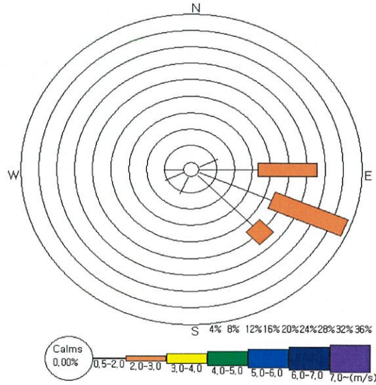
그림 2. 서구지역 바람장미
